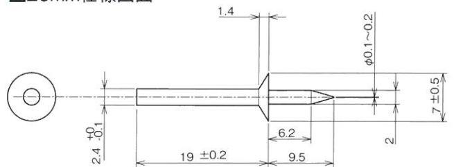
■20mm仕様図面
