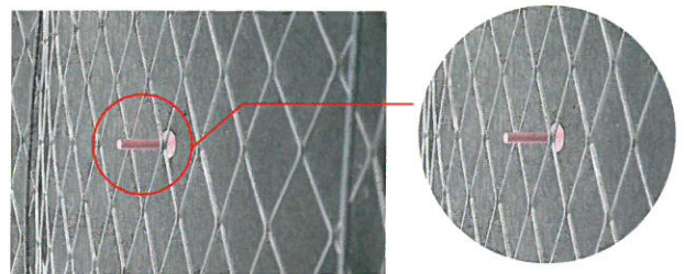
下地パネルにモルきんくんの底部の針で固定する。 (手で押し込めない場合はハンマー等で打ってください)
