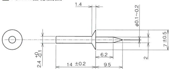
■15mm仕様図面
